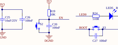
MCU部分 带WiFi功能
