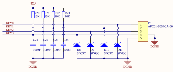
按键输入部分
