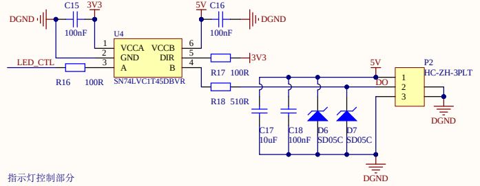
指示灯控制部分
